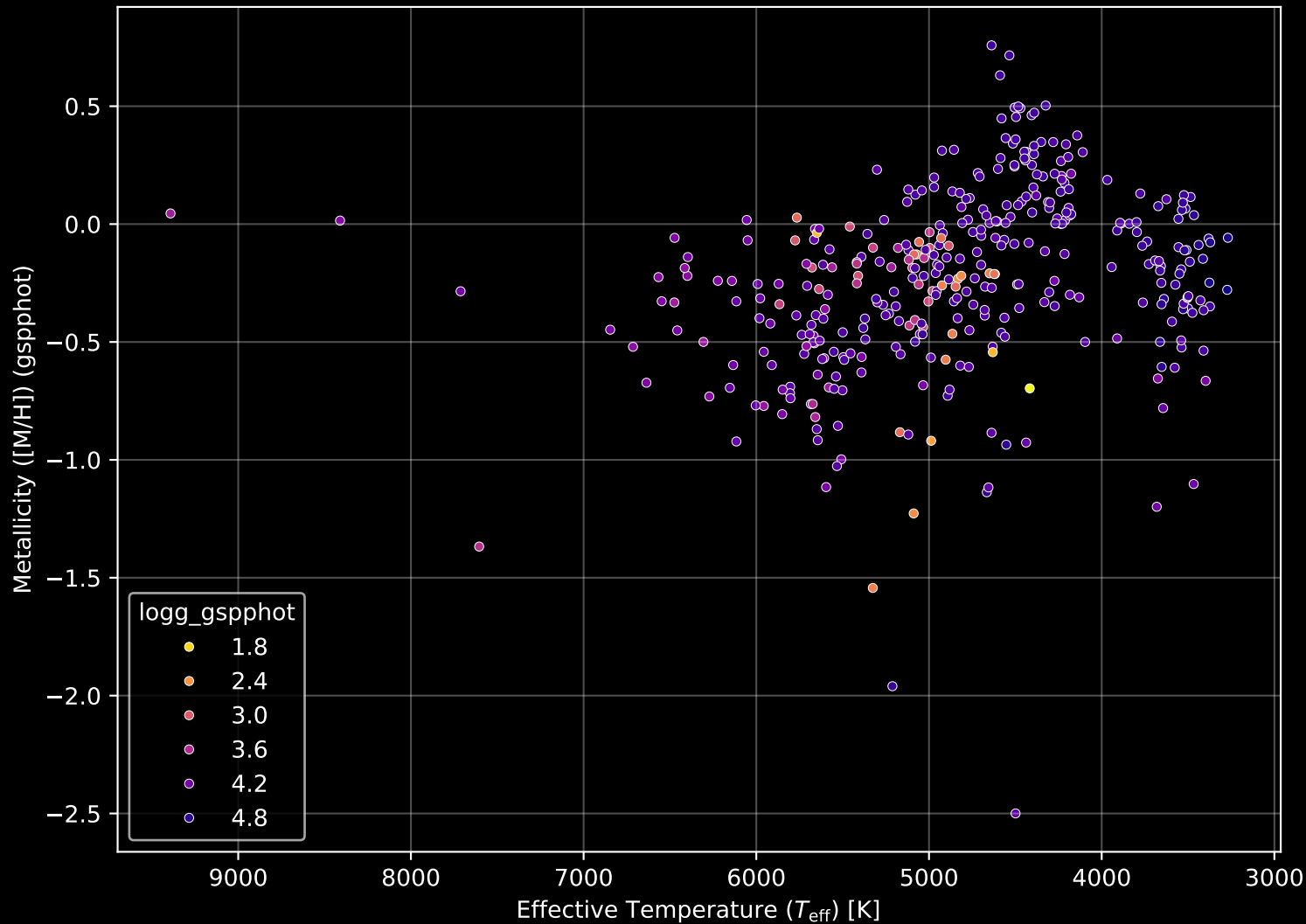
APOGEE DR17 Field: [120+75] Stellar Population Parameters (n= 372)
